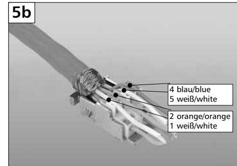
5b ... die Adernpaare blau/weiß und orange/weiß oben in das Ladestück einlegen. ... and the wire pairs blue/white and orange/white in the upper wire guides of the loader.
