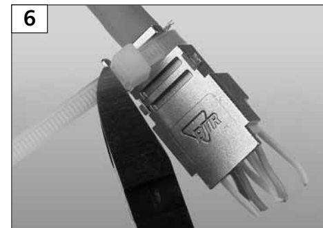
6 Kabelbinder zur Zugentlastung anbringen und Überlänge entsprechend abschneiden. Fit a cable tie and cut off the excess length.
