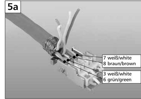
5a Die Adernpaare weiß/braun und weiß/grün in die unteren Öffnungen des Ladestücks einführen ... Insert the wire pairs white/brown and white/green in the lower wire guides of the loader ...
