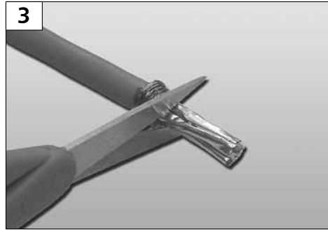
3 Paar-Schirmfolie einkerben und entfernen. Cut and remove the shield foil of the wire pairs.
