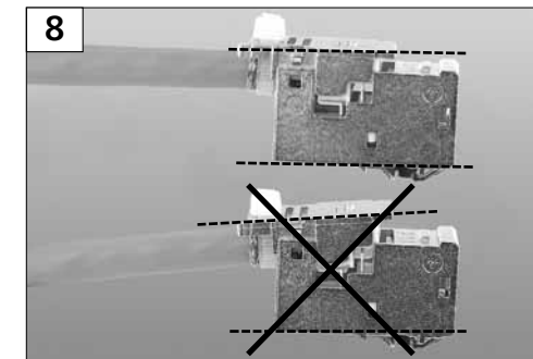
8 Beim Zusammenfügen der Gehäuseteile, das Ladestück gerade auf das Gehäuseunterteil setzen. When the two housing parts are assembled make sure that the loader is correctly aligned with the lower housing.
